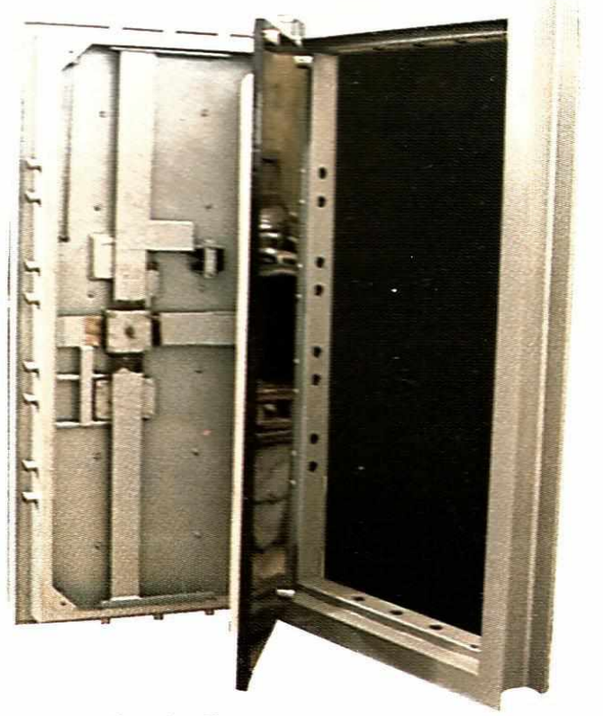
Açık Oda Kapısı OK. 606
